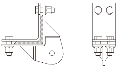
耐张夹板 Tensile clamp
