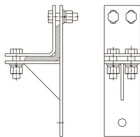
直线夹板 Straight line clamp
