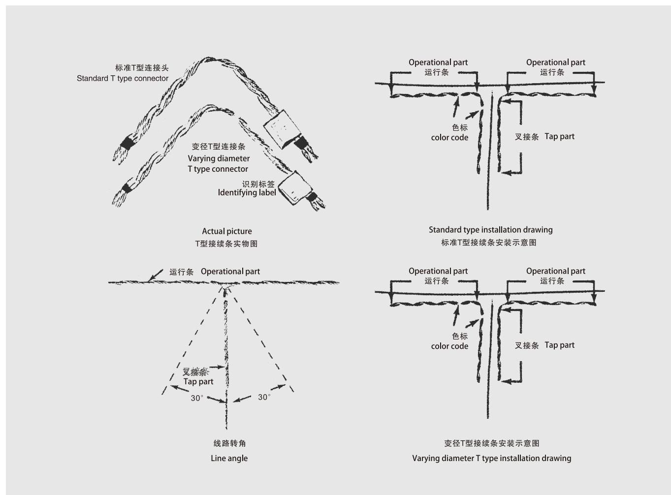
图Drawing 6-6
